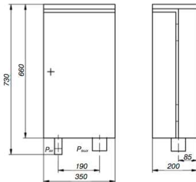
Габаритный чертеж
