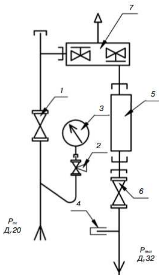
Схема пневматическая функциональная «ГРПШ/ГРУ-10(25)-1-СГ» :
