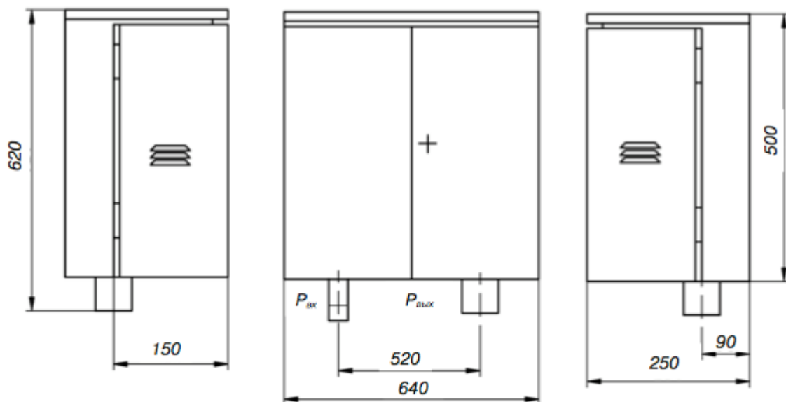
Габаритный чертеж
